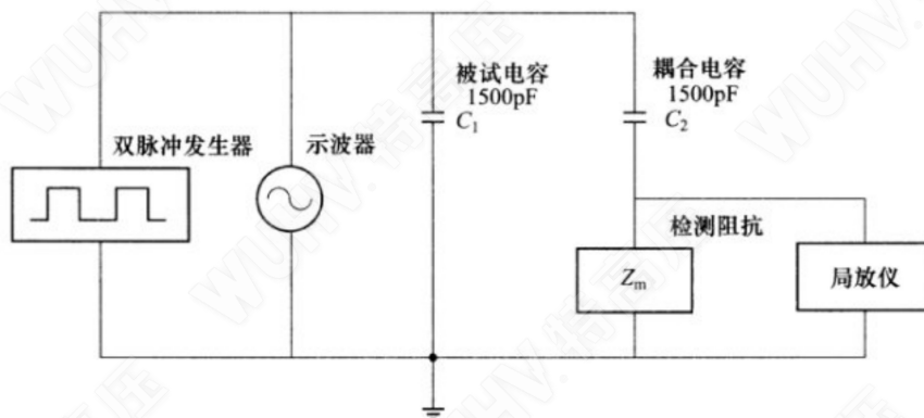
图 3 脉冲分辨时间的误差校准接线图
