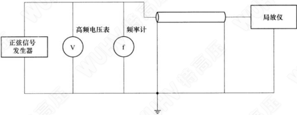
图 1 频带与截止频率试验接线图
