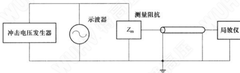
图5 测量阻抗过电压保护性能试验接线图
