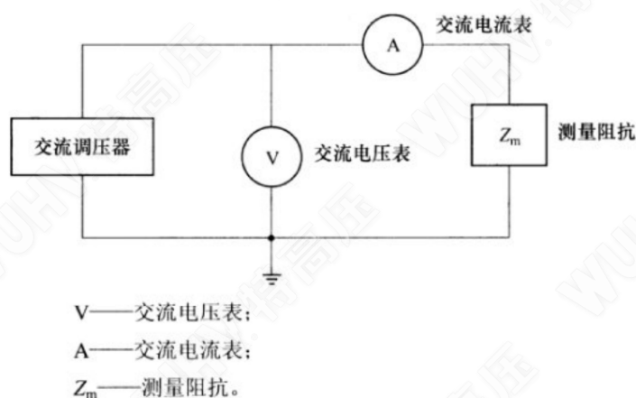
图 4 测量阻抗通流能力试验接线图
