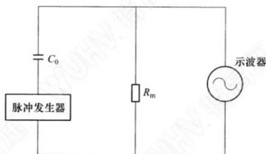
图 A.1 电荷量积分算法试验接线图
