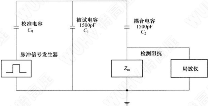
图 2 线性误差试验接线图
