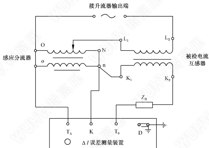
图 6 感应分流器检定电流互感器线路
