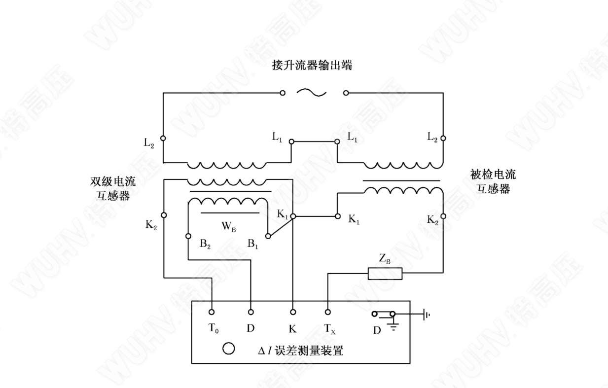
图 3 双级电流互感器检定电流互感器线路
