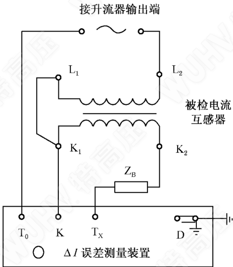
图 1 电流互感器自检线路
