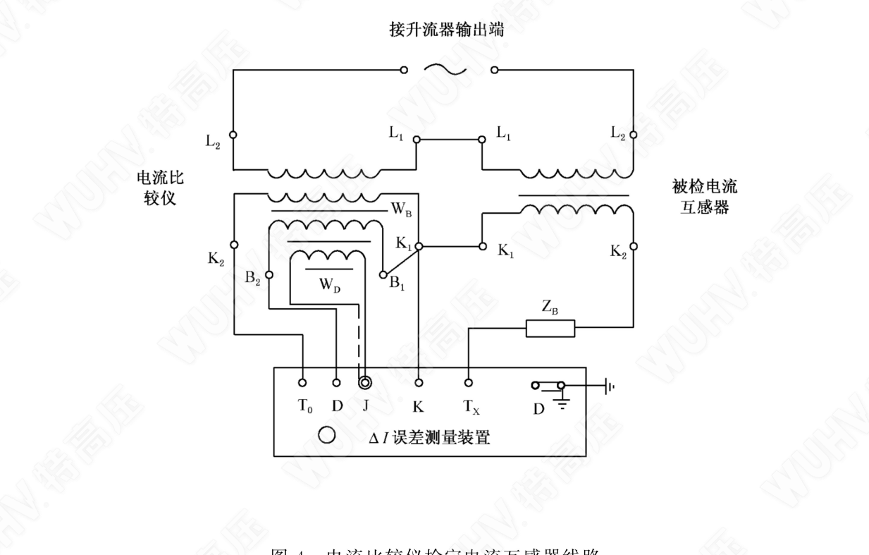
图 4 电流比较仪检定电流互感器线路
